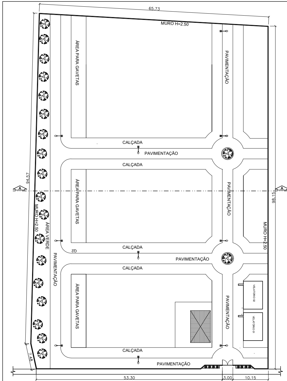
1 PLANTA BAIXA esc 1:500
